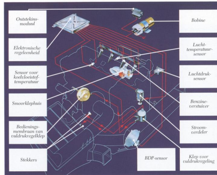
Elektronisch motorregelsysteem
