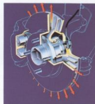
Geventileerde remschijf met elektromagnetische sensor van ABS-systeem
