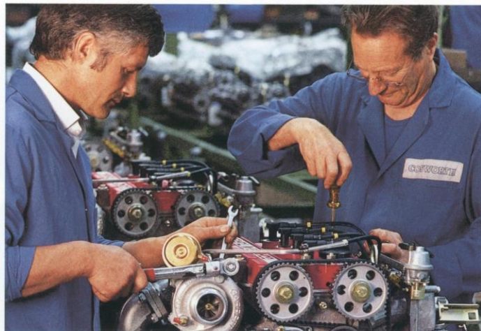
Handmatige eindmontage van Cosworth motor
