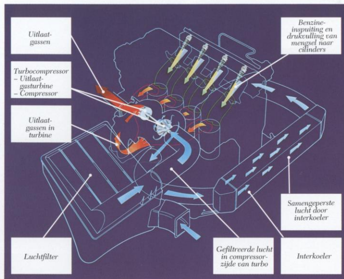
Schema van de drukvulling d.m.v. een turbocompressor
