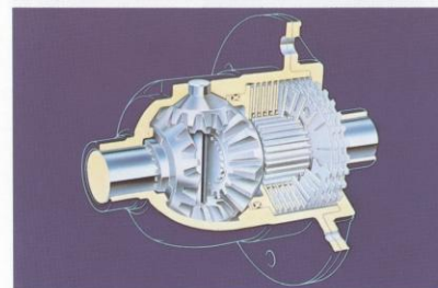
Zelfblokkerend differentieel met viscokoppeling
