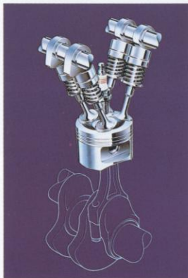
Verbrandingskamer met vier kleppen
